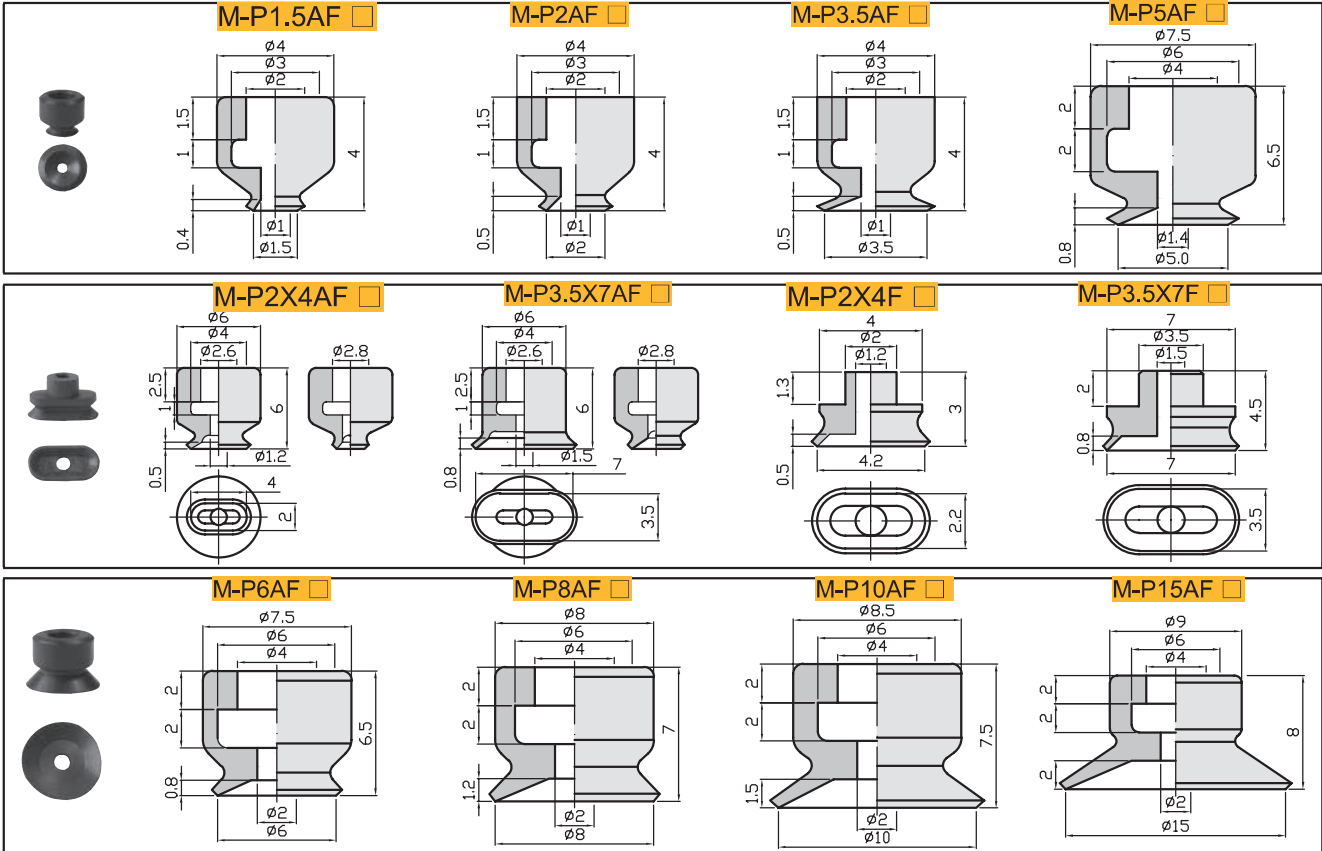
外形尺寸图 注：“★”为畅销规格，库存充足。
