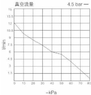
不同真空度 (-kPa) 的真空流量 (l/min)
